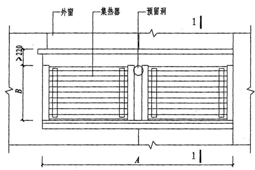
立面图
