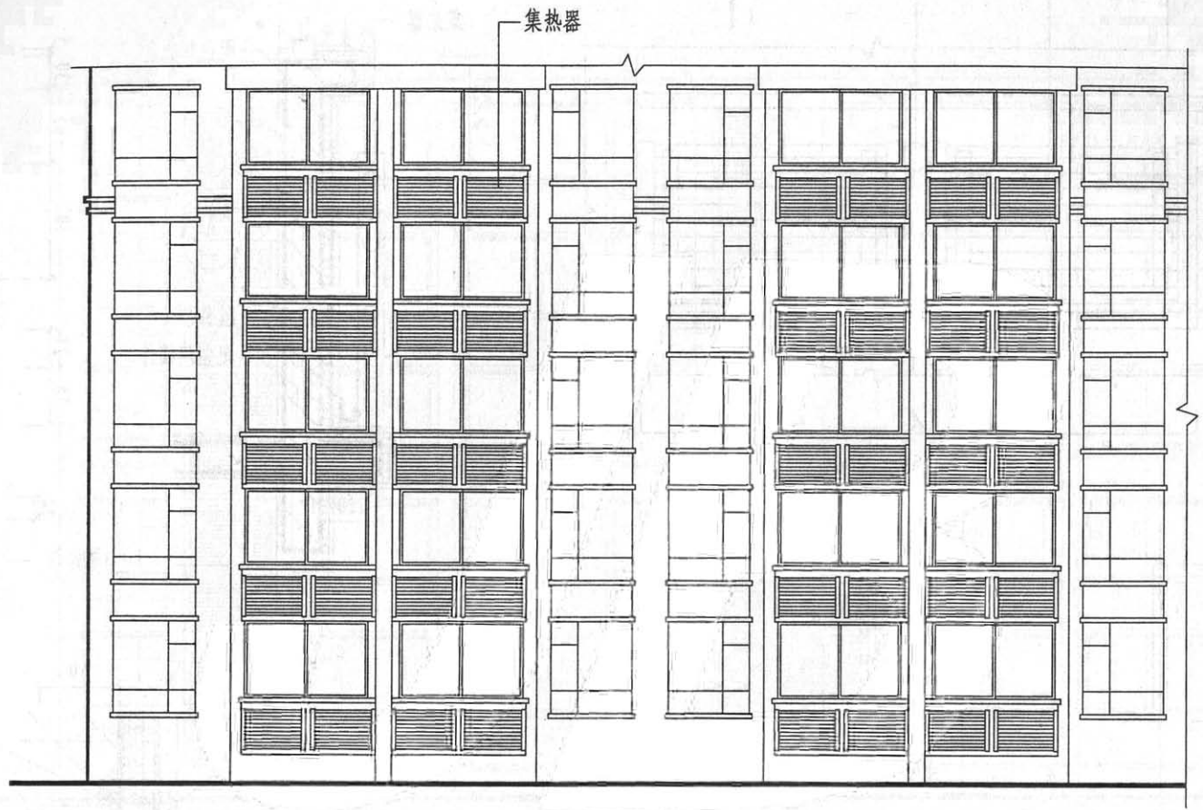
立面布置示例
