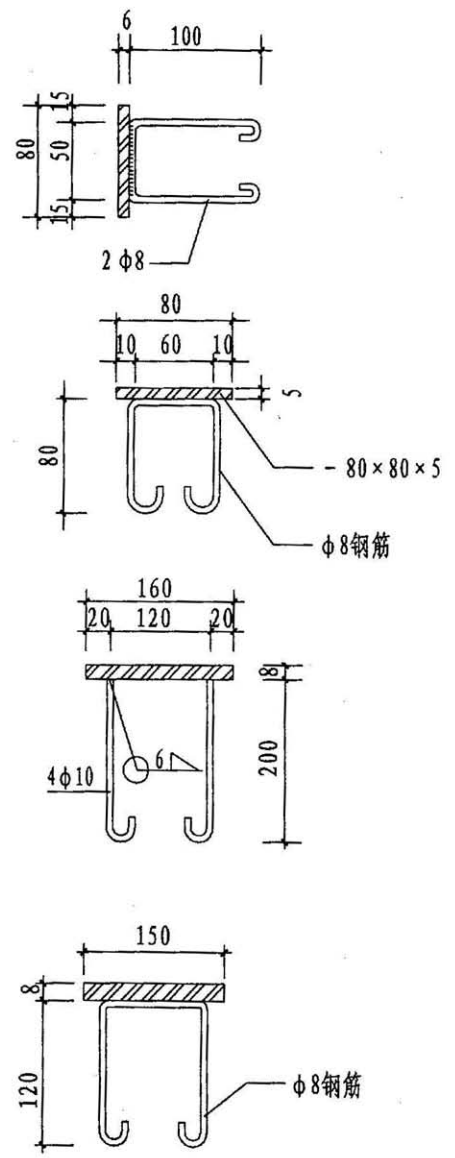
预留支座详图、预埋件详图
