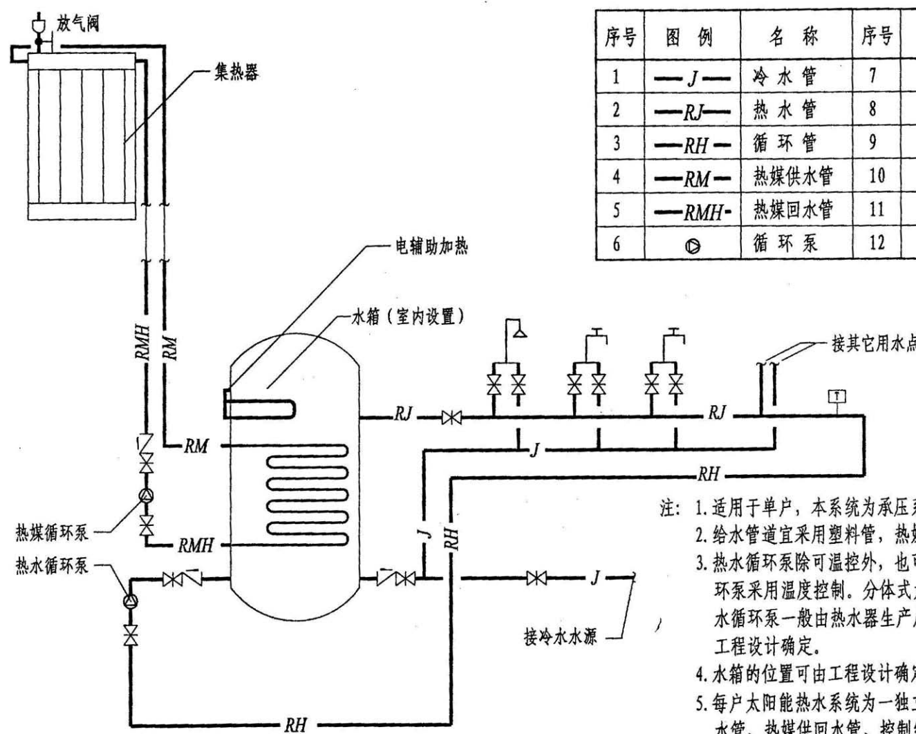
分体承压式原理图
