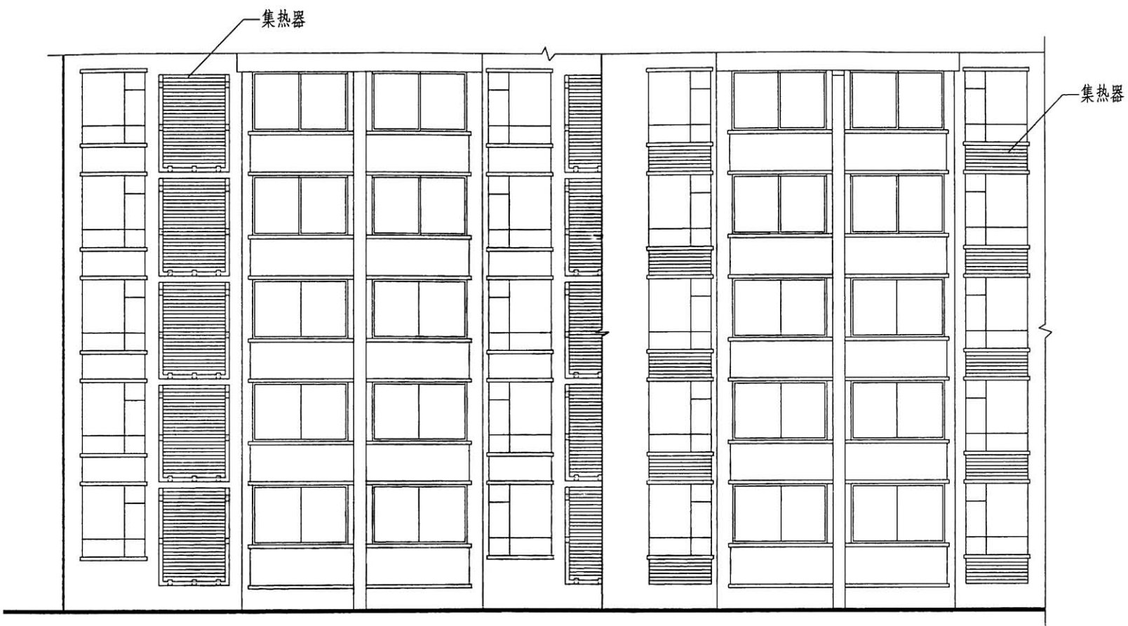
立面布置示例
