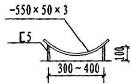
水箱托架
