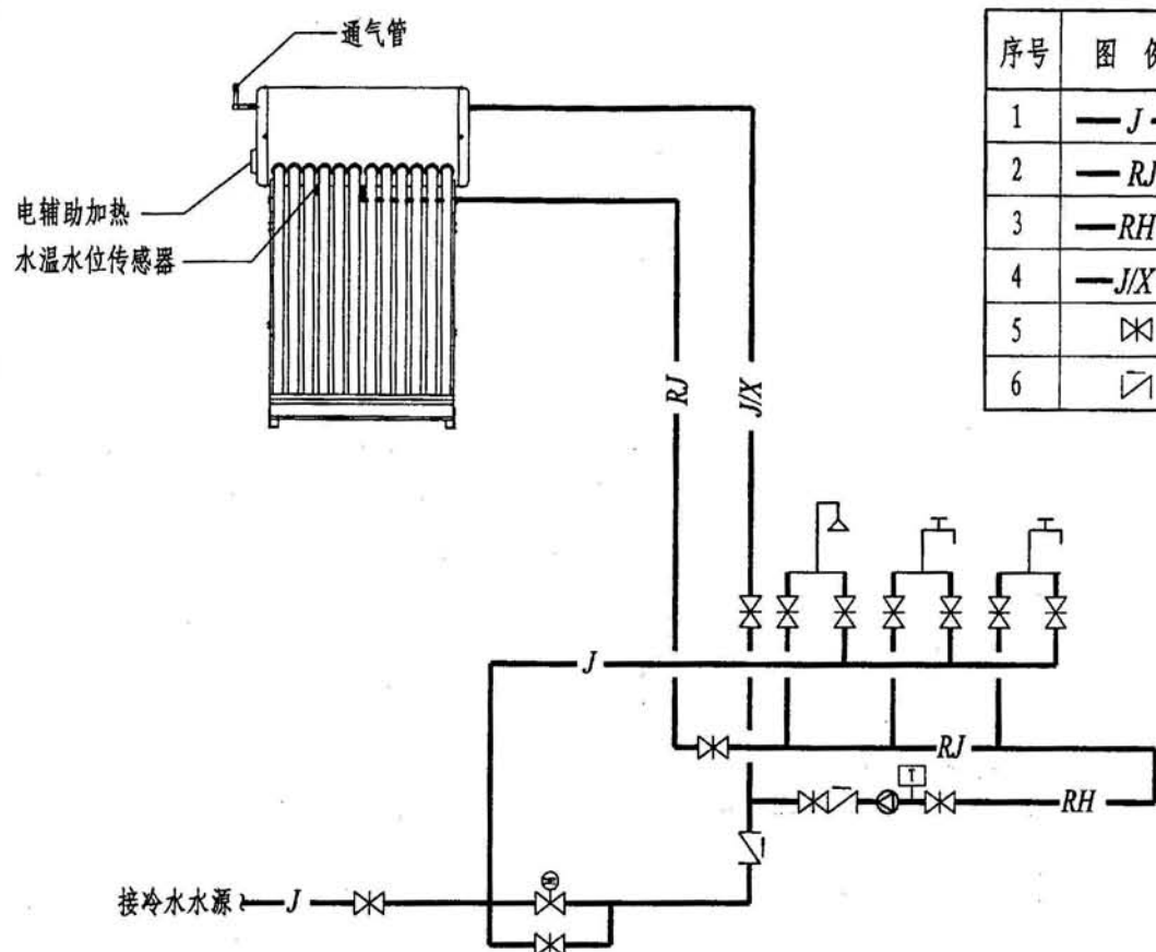
双管整体式太阳能热水器原理图
