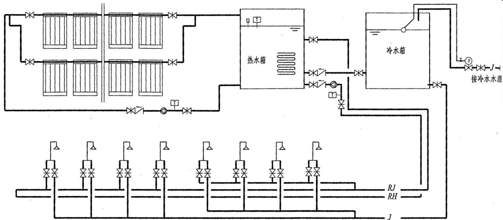
集中热水双管系统
