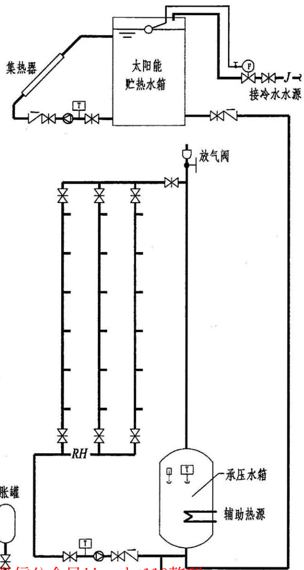
强制循环双水箱直接系统
