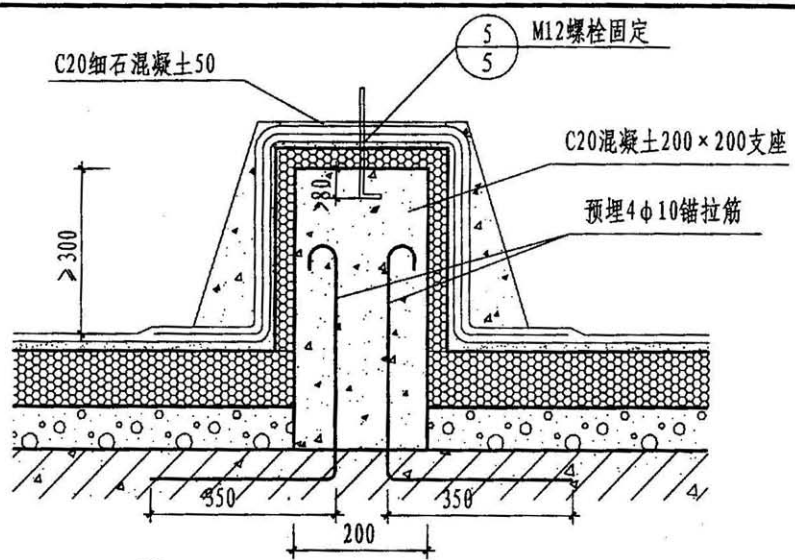
① 有保温屋面
