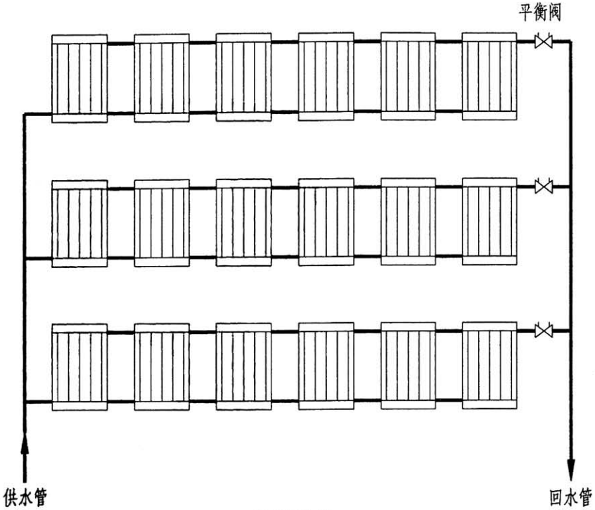
b 异程连接
