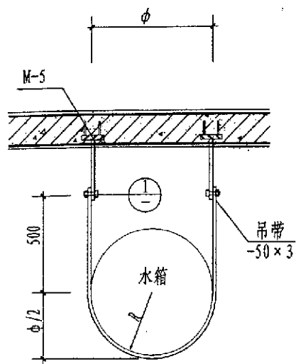
平屋顶水箱吊装图
