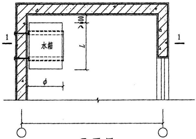
平面图
