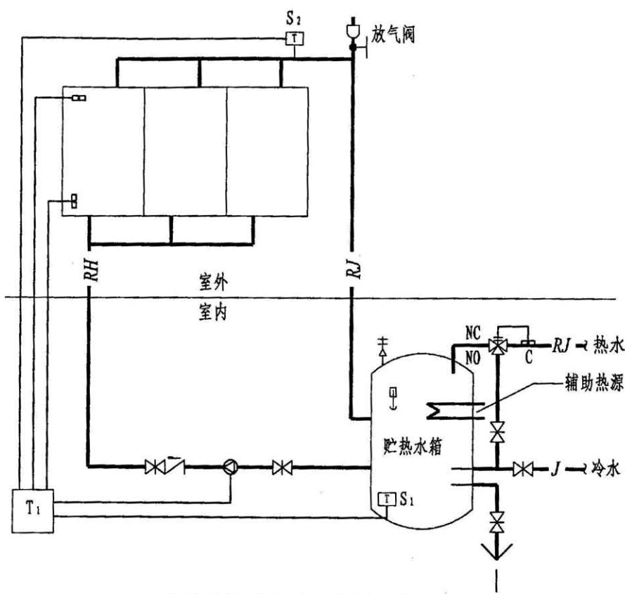
直接系统温差循环控制系统
