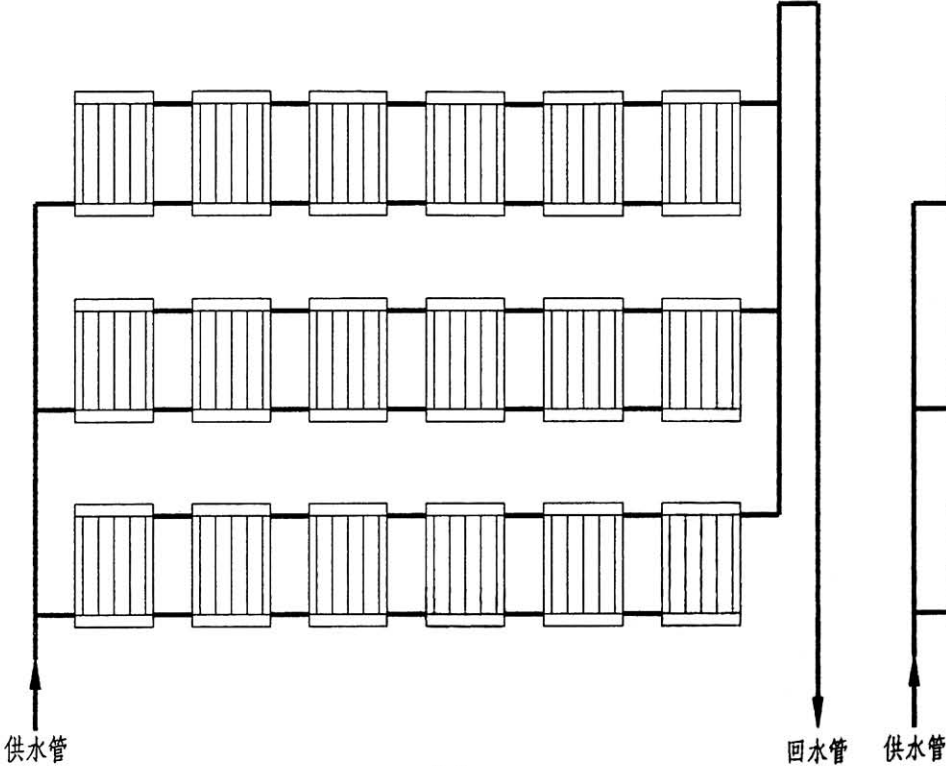
a 同程连接
